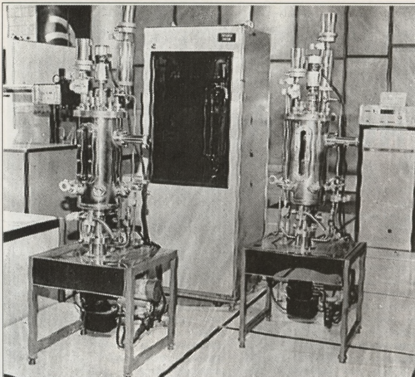
Одна из разработок НИИ биотехники: ультрафильтрационная универсальная установка
