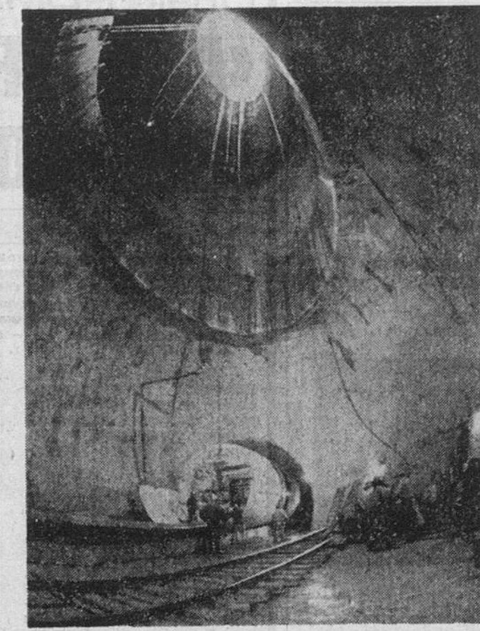
Президент США Клинтон энергично выступил за финансирование создания сверхускорителя. Он отметил, что роль этого ускорителя в развитии самых современных технологий чрезвычайно важна. В штате Техас сооружен первый туннель сверхускорителя, подземная труба длиной в 54 мили, где атомы будут разогнаны на очень высокой скорости, а затем расщеплять.
