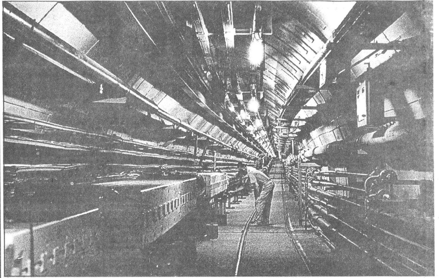
В подземном тоннеле расположено важное звено протонного синхротрона — канал инжекции протонов.
