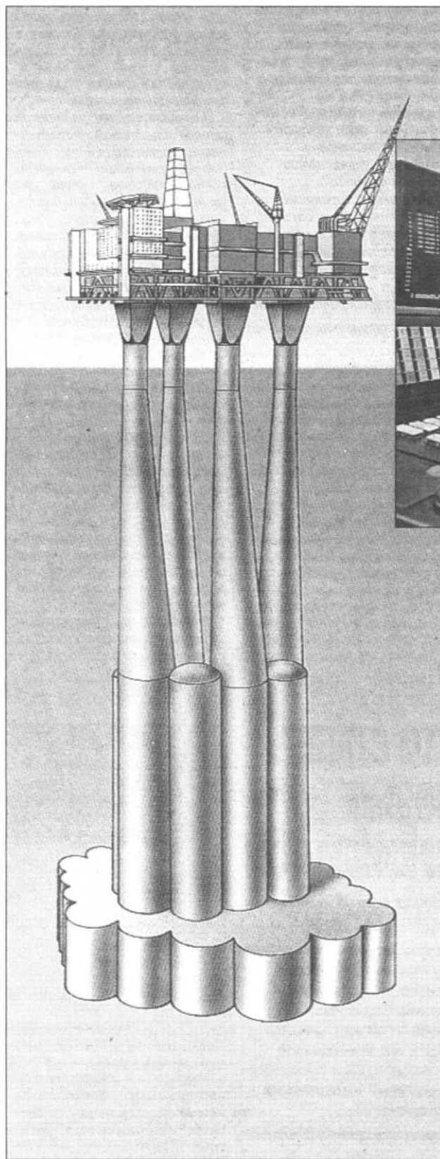
Глубина под водой — около 350 метров, общая высота — около 470 метров. Модель одной из установок
