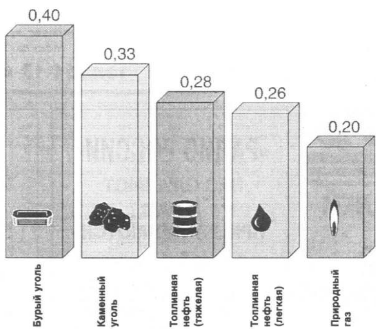
Образование CO 2 при сгорании сжигаемых источников энергии (в кг CO 2 на кВт/ч топлива)
