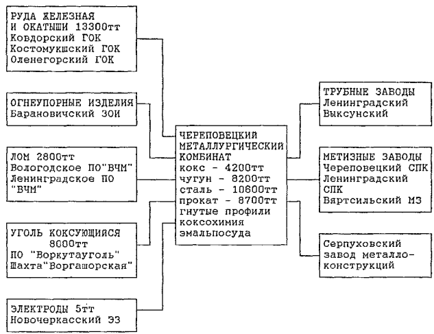
Принципиальная схема
